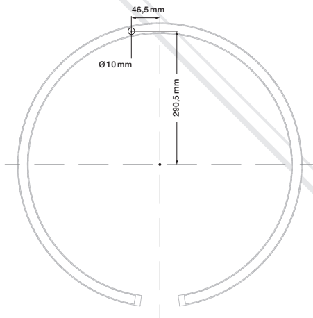
Abb. zeigt die empfohlene Ausrichtung der Leuchte. Figure shows the recommended orientation of the luminaire.
